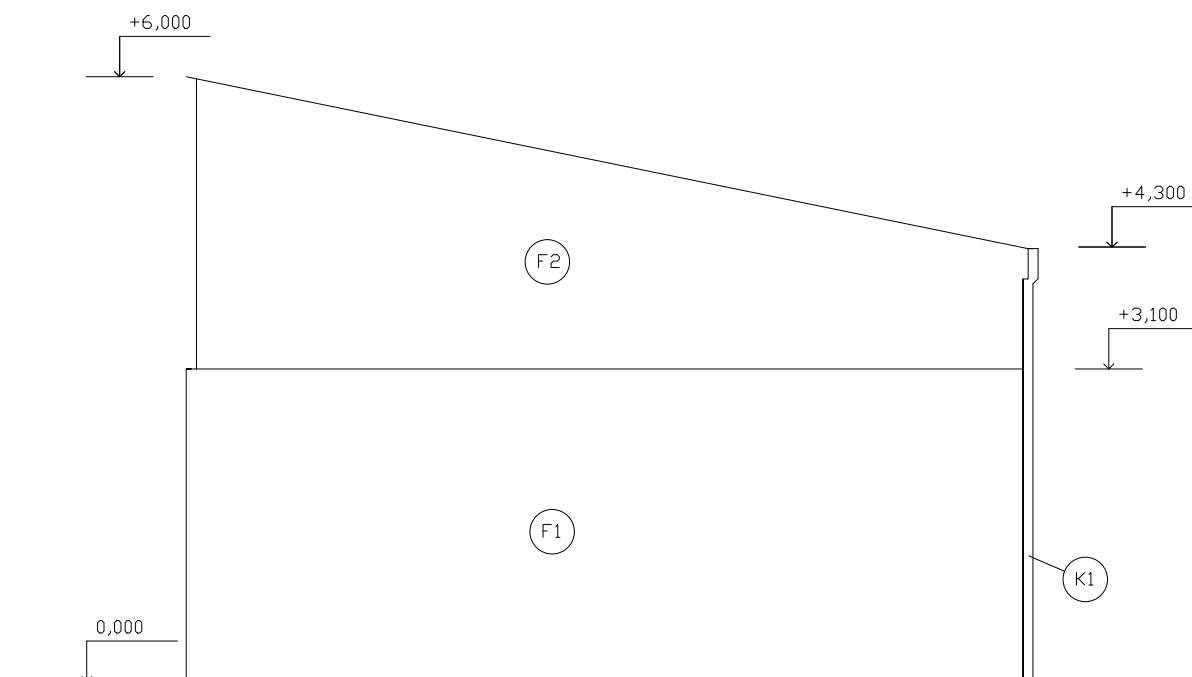
POHLAD ZÁPADNÝ
