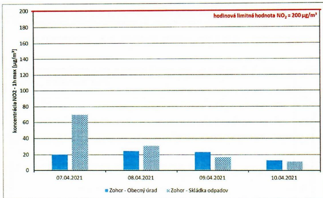
Obrázok 7: Maximálne hodinové hodnoty koncentrácií NO 2
