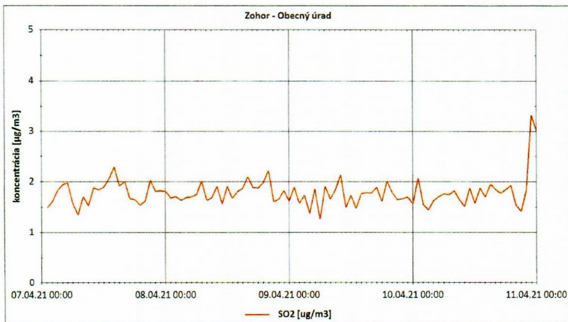
Obrázok 1: Priemerné hodinové koncentrácie SO 2 , Zohor – Obecný úrad
