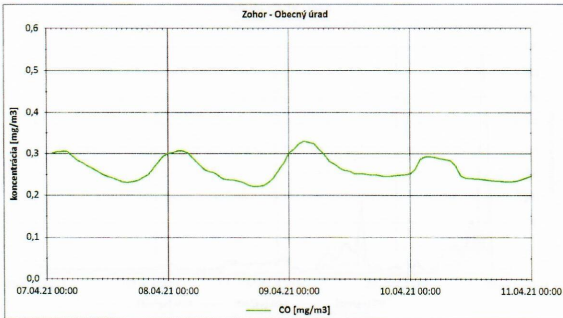
Obrázok 3: Priemerné 8- hodinové koncentrácie CO, Zohor – Obecný úrad
