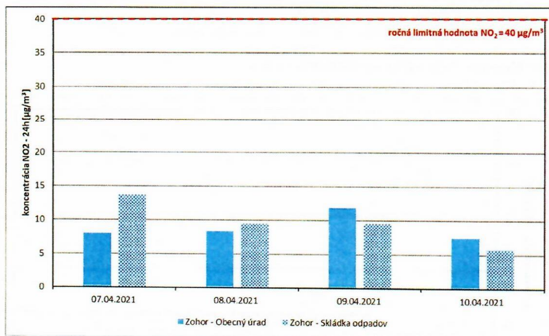
Obrázok 8: Priemerné denné hodnoty koncentrácií NO 2
