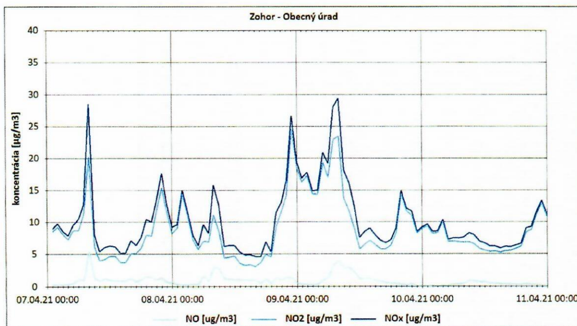
Obrázok 2: Priemerné hodinové koncentrácie NO 2 – NO x , Zohor – Obecný úrad
