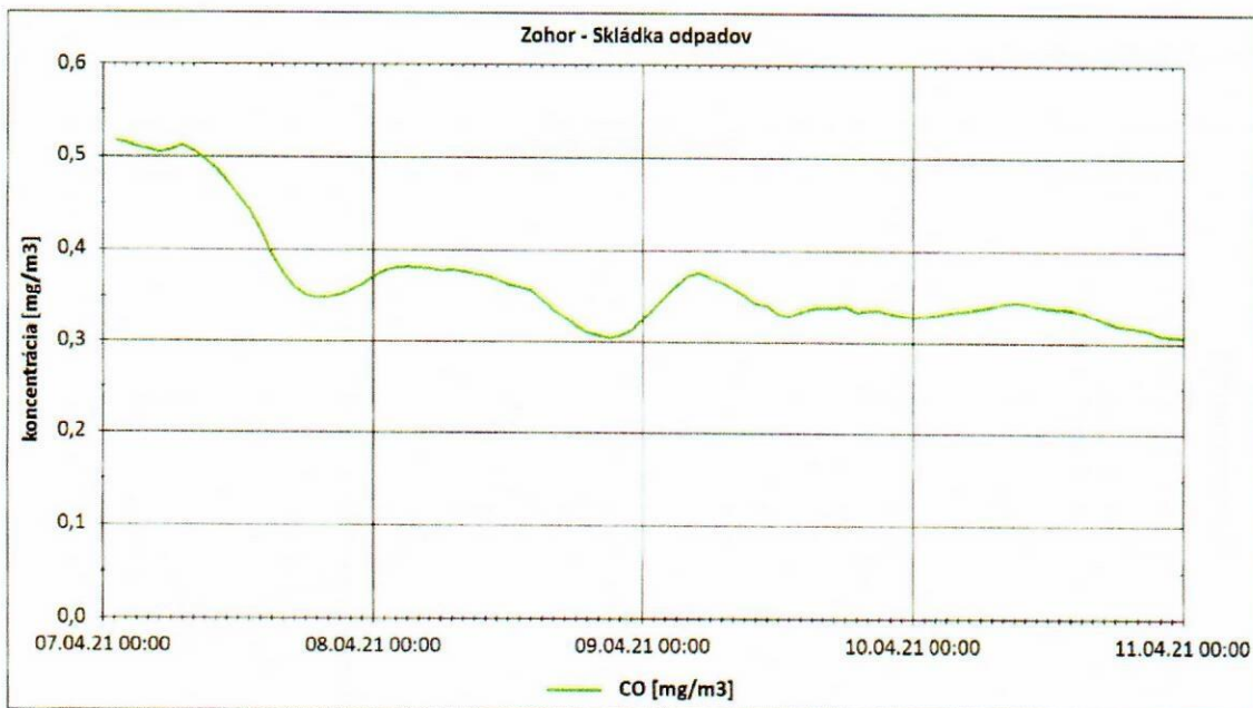
Obrázok 6: Priemerné 8- hodinové koncentrácie CO, Skládka odpadov
