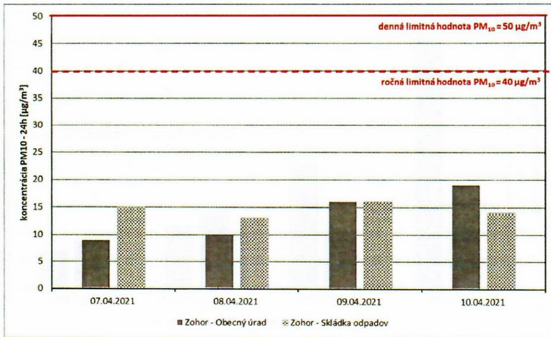
Obrázok 11: Priemerné denné hodnoty koncentrácií PM 10
