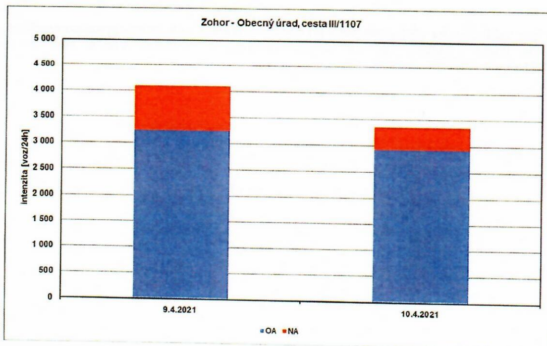
Obrázok 14: Zloženie a intenzita dopravy v reze komunikácie III/1107 1)
