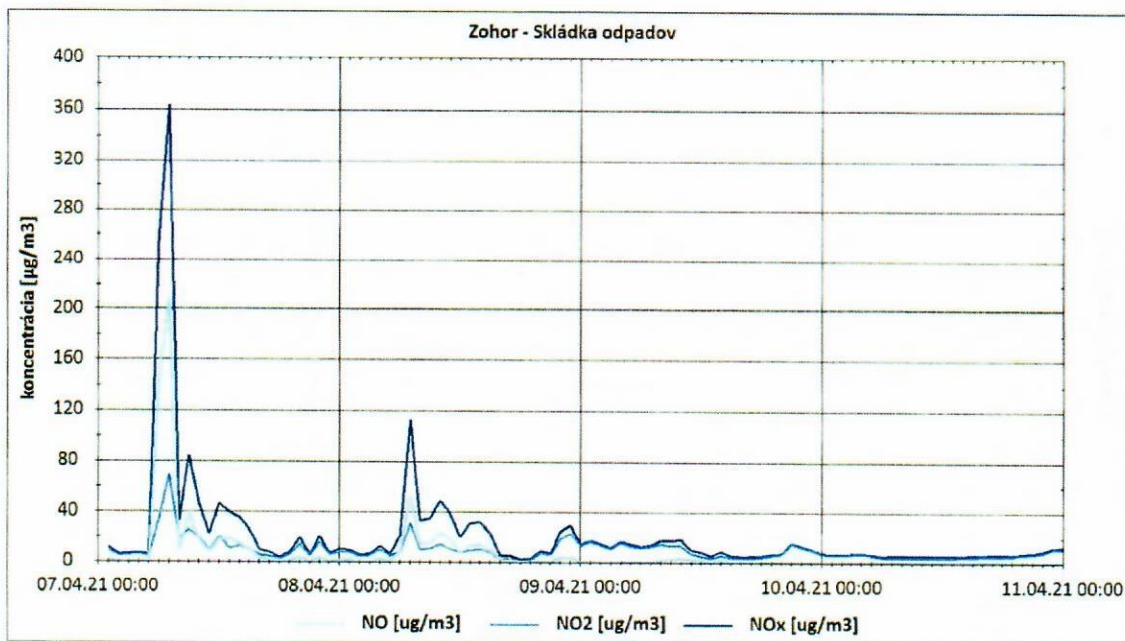
Obrázok 5: Priemerné hodinové koncentrácie \text{NO}_2 - \text{NO}_x , Skládka odpadov
