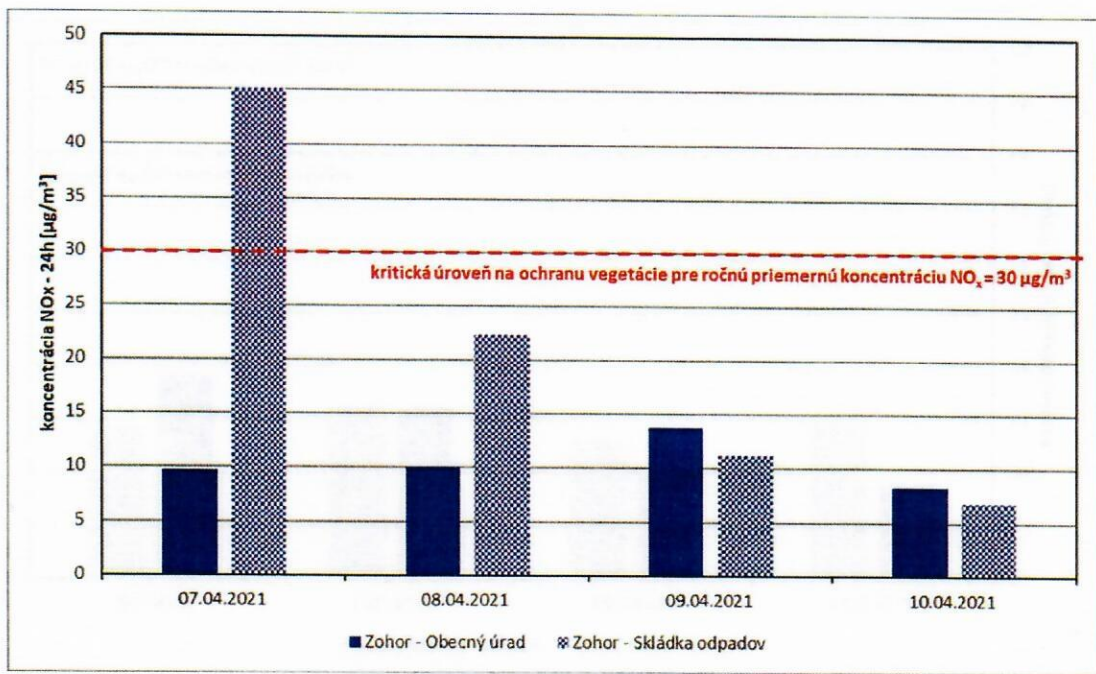
Obrázok 9: Priemerné denné hodnoty koncentrácií NO x
