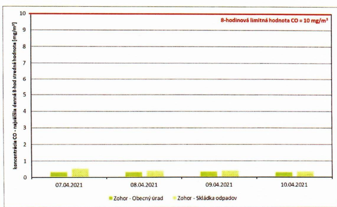
Obrázok 10: Najväčšie denné 8- hodinové stredné hodnoty koncentrácií CO
